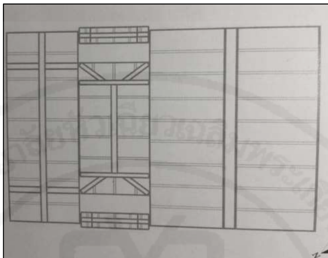
ภาพที่ 6 ผังหลังคาของศาลเจ้ากวนอู (ตลาดสมเด็จพระยา) ใช้รูปอักษรจีน“工” (GONG)
